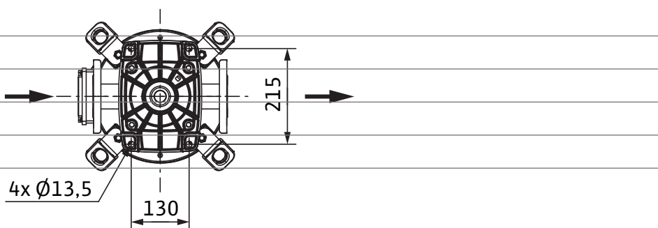
Габаритный чертеж
